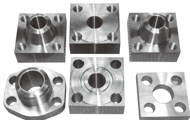
高圧フランジ(規格、ユーザー仕様他)
