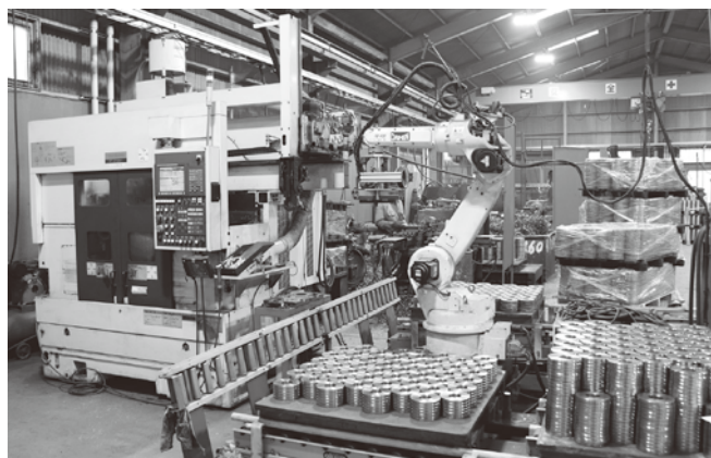
ロボット付CNC旋盤
