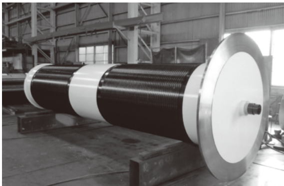
コンテナクレーン用ドラムφ1900×6000mm
